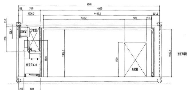
A-A 矢視
