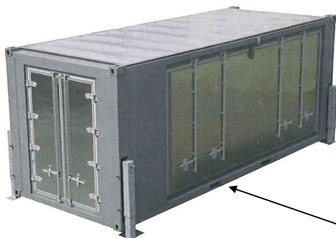
◎移送時外観
